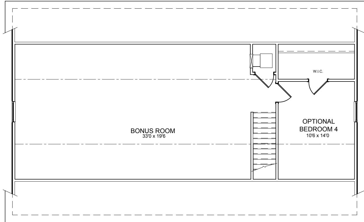
OPTIONAL BEDROOM 4 PLAN
