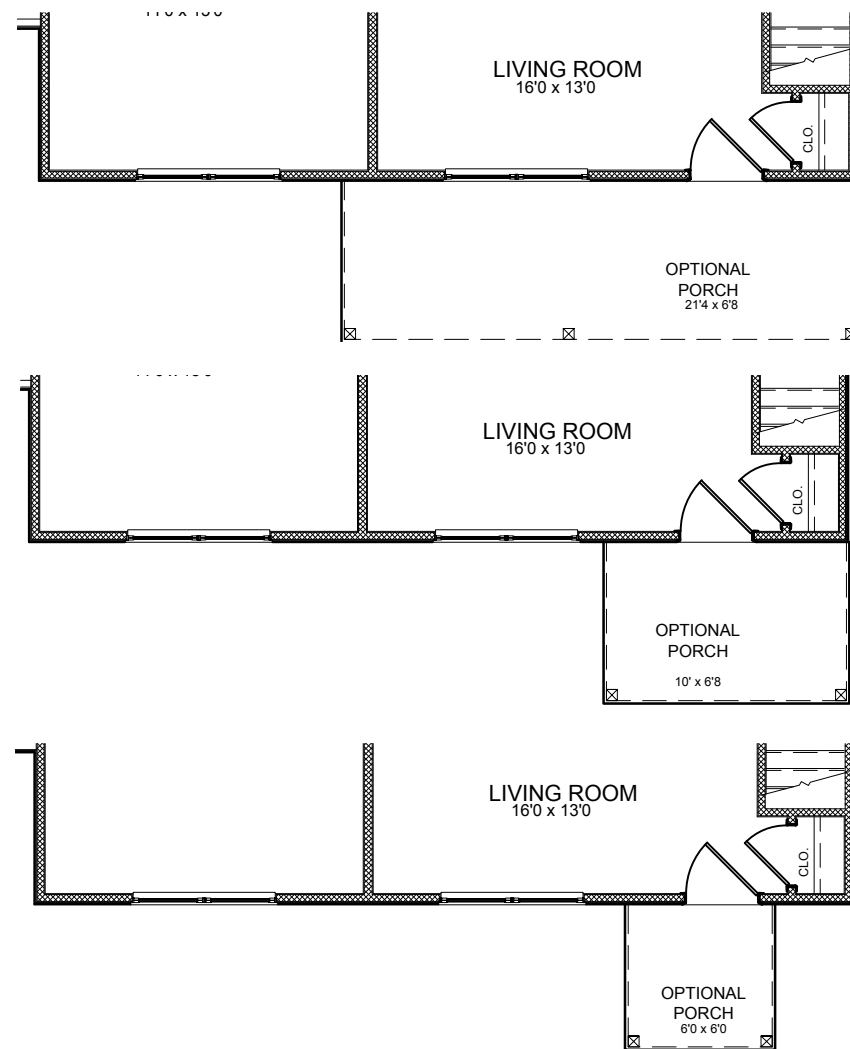
PORCH OPTIONS
