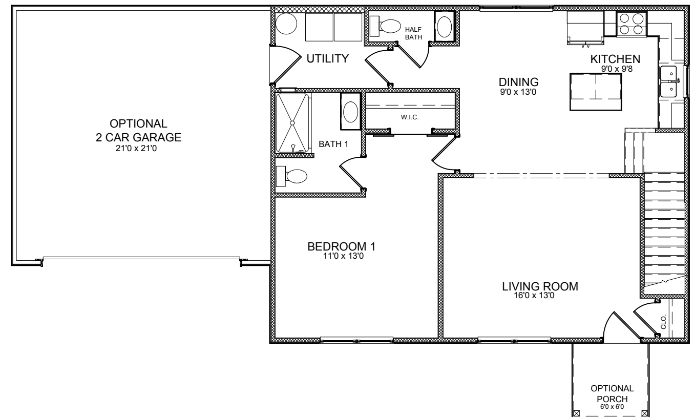
OPTIONAL GARAGE PLAN
