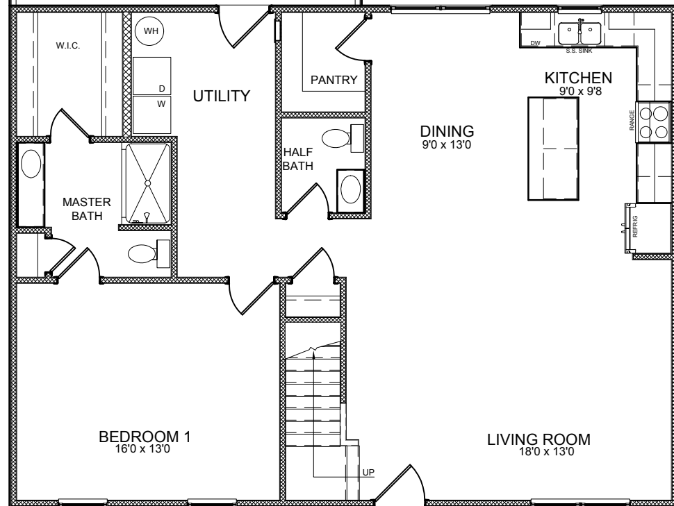
OPTIONAL GARAGE
